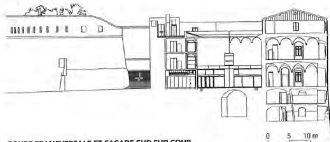
COUPE TRANSVERSALE ET FAÇADE SUD SUR COUR
