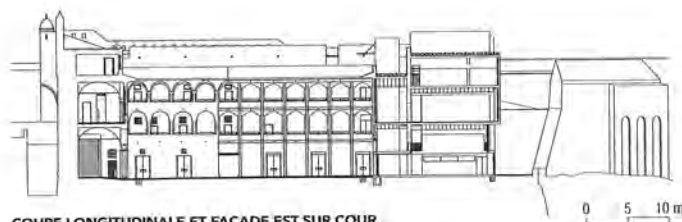
COUPE LONGITUDINALE ET FAÇADE EST SUR COUR
